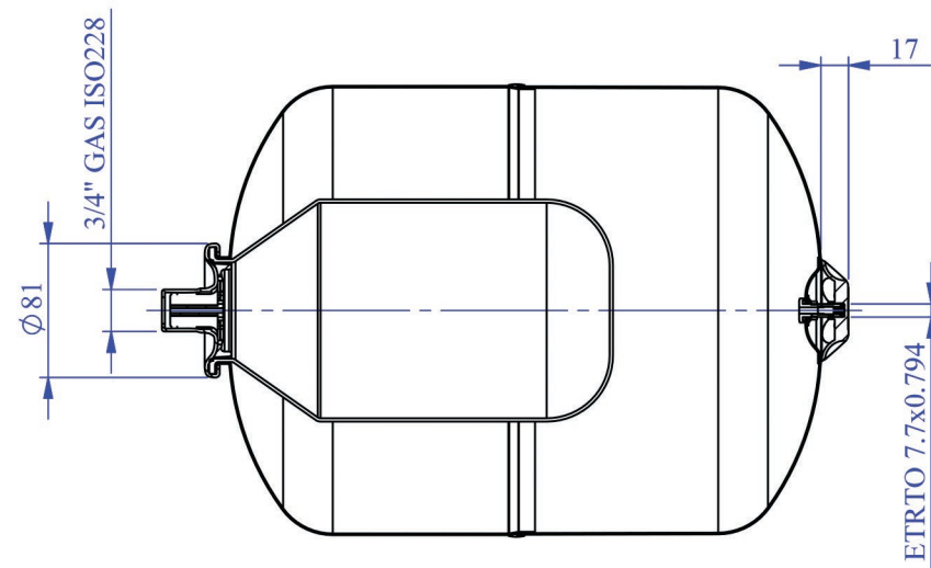
SEZIONE A-A
